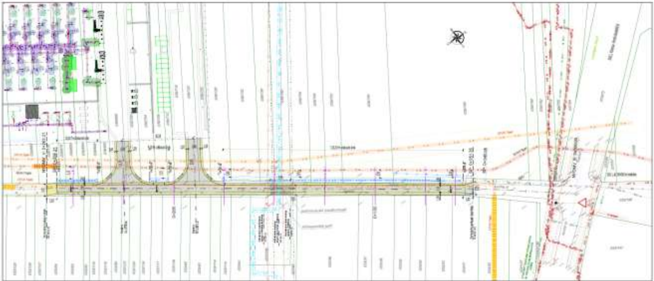
Forrás: Útépítés és vízelvezetés kiviteli terve (Chess Energy Kft. 2026.) 3101. számú (Új Ecseri út) csomópont tervezett átépülése
