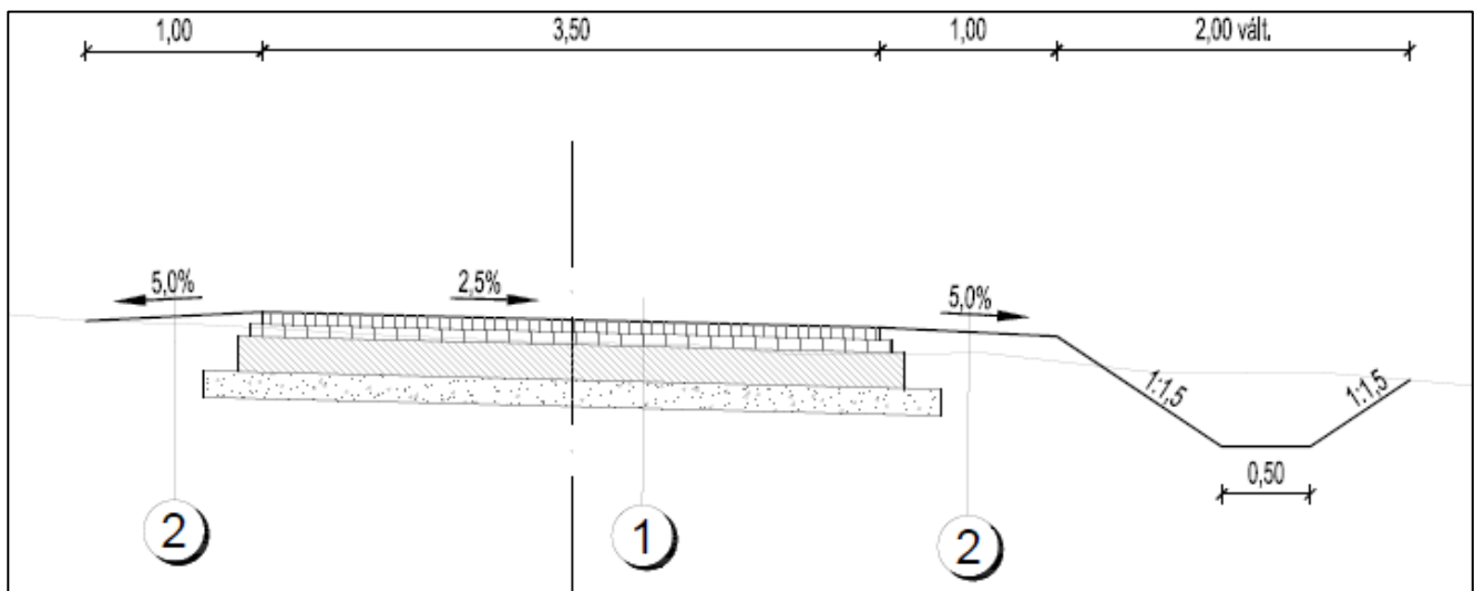
Forrás: Jellemző mintakeresztmetszvény (Chess Energy Kft. 2026.) 3101. számú (Új Ecseri út) csomópont tervezett átépülése
