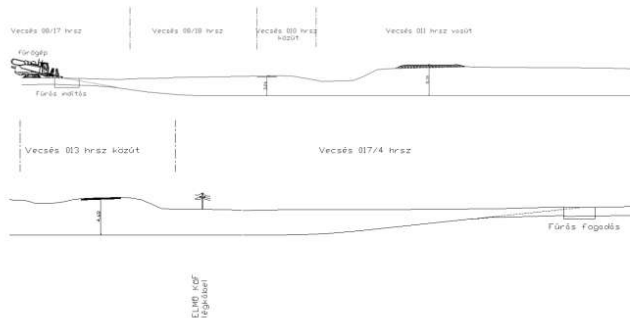
18. ábra: Mélyfúrással érintett vezetékfektetés Forrás: Senex Környezetgazdálkodási Kft.: Előzetes vizsgálati dokumentáció-2025.01.
